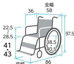
自走 中床 (NEXT-71B)
